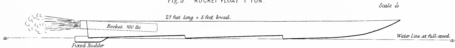
Fig. 3. ROCKET FLOAT 1 TON.
